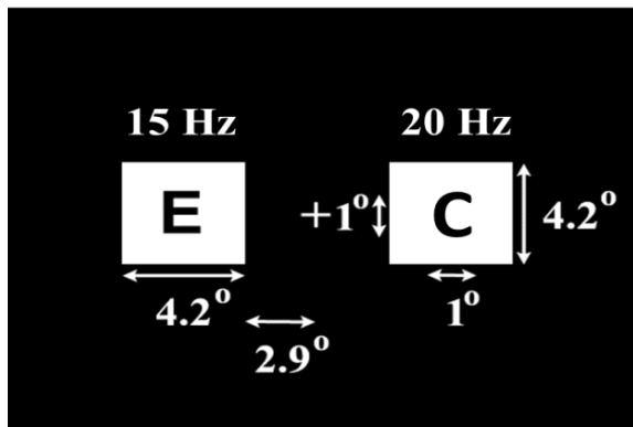
Fig. 1. Stimulus Display
